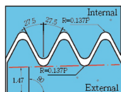
BSPT 55° 英制錐管螺紋 55°
