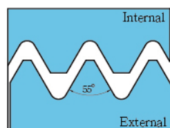
Partial Profile 55° 通用螺紋 55°
